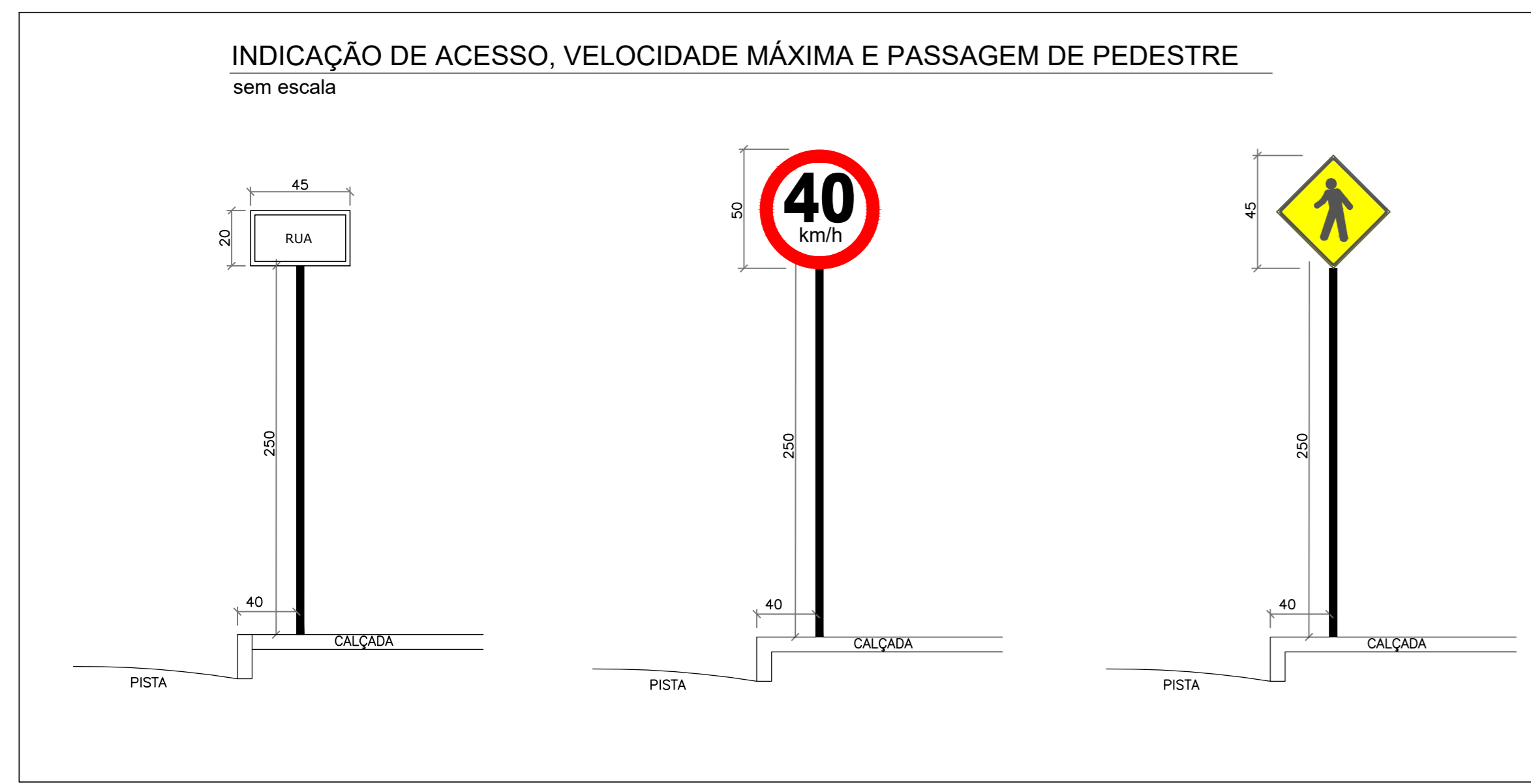
Det. 08 - Sinalização vertical Sem escala
