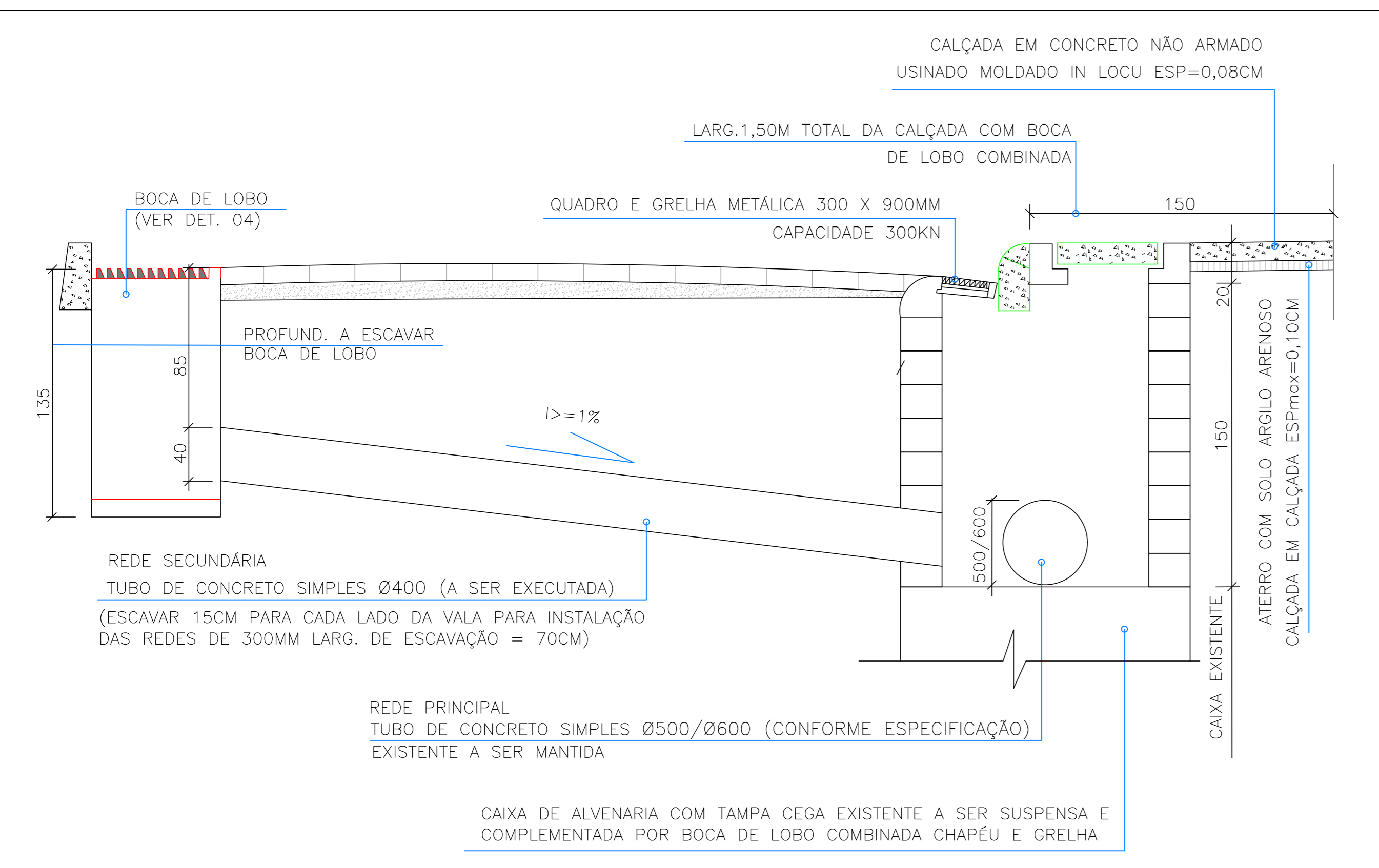
Seção transversal de drenagem Sem escala
